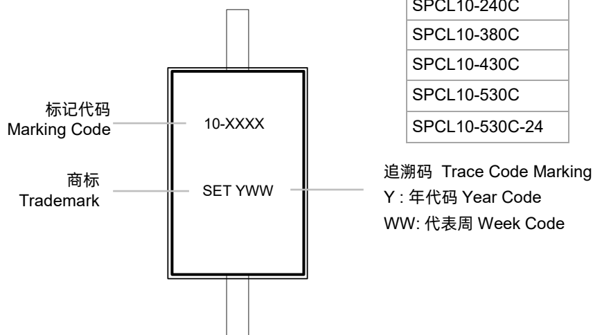
类型2 - 俯视图 Type 2 - Top View
