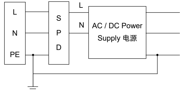
串联（两端口） Series Connection (Two-port)
