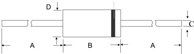
DO - 201
