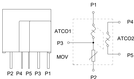
TFMOV(ATCO) 热保护型压敏电阻（熔断合金型）
