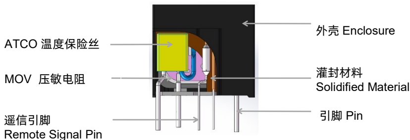
TFMOV(ATCO) 热保护型压敏电阻（熔断合金型）
