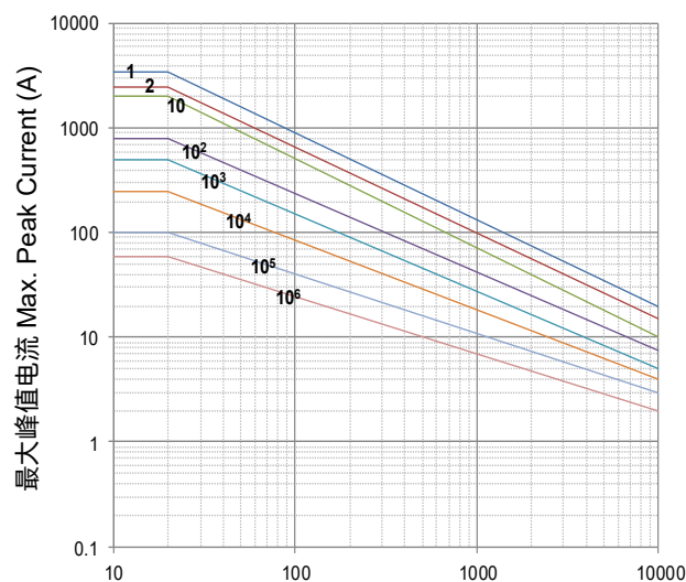
脉冲持续时间 Impulse Duration ( \mu s) SFV10D820KT to SFV10D122KT
