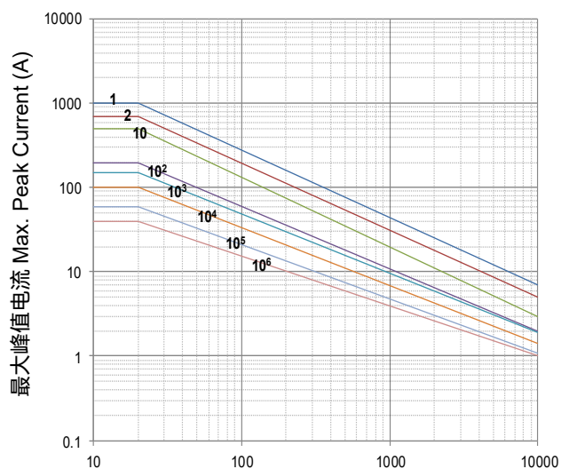
脉冲持续时间 Impulse Duration ( \mu s) SFV10D220KT to SFV10D680KT
