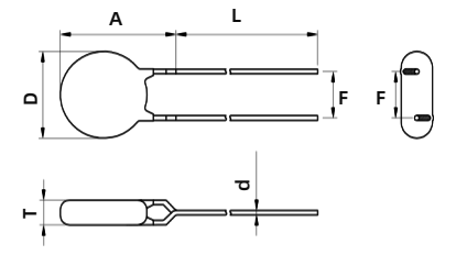
Y型引线 Inline Crimp
