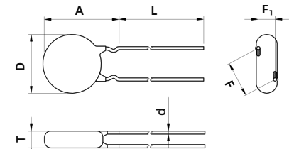
内弯型引线 Inward Crimp
