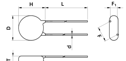
直型引线 Straight Lead
