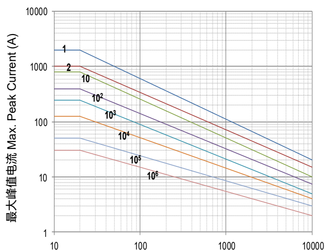
脉冲持续时间 Impulse Duration ( \mu s) SFV14D220KT to SFV14D680KT
