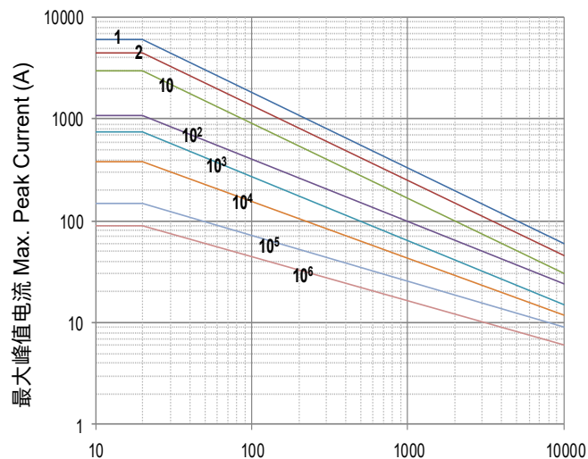
脉冲持续时间 Impulse Duration ( \mu s) SFV14D820KT to SFV14D122KT
