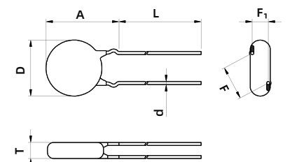
外弯型引线 Outward Crimp
