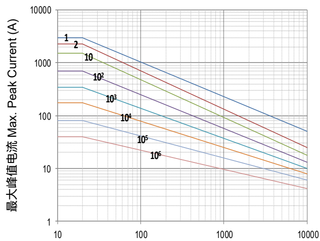
脉冲持续时间 Impulse Duration (μs) SFV15S220K to SFV15S680K
