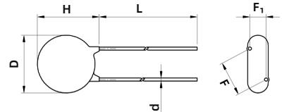
直型引线 Straight Lead
