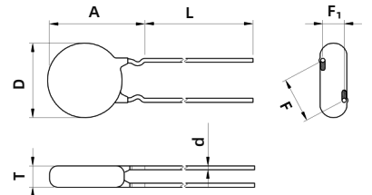
内弯型引线 Inward Crimp
