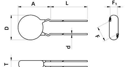
外弯型引线 Outward Crimp
