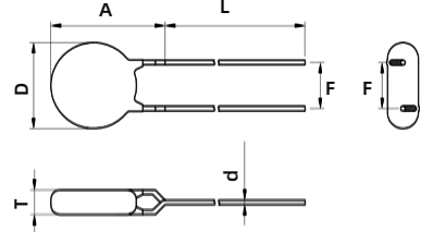
Y型引线 Inline Crimp
