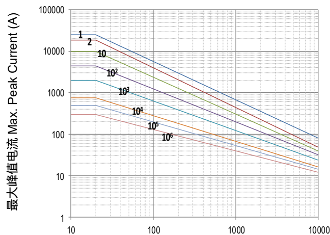
脉冲持续时间 Impulse Duration ( \mu s) SFV25S820K to SFV25S122K
