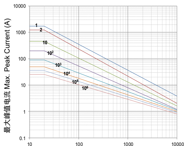
脉冲持续时间 Impulse Duration ( \mu s) SFV7D820KT to SFV7D821KT
