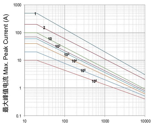
脉冲持续时间 Impulse Duration ( \mu s) SFV7D220KT to SFV7D680KT
