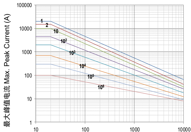
脉冲持续时间 Impulse Duration ( \mu s) SFV25D820KM to SFV25D122KM
