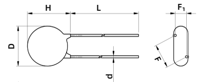
直型引线 Straight Lead
