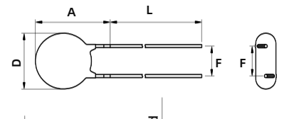
外弯型引线 Outward Crimp
