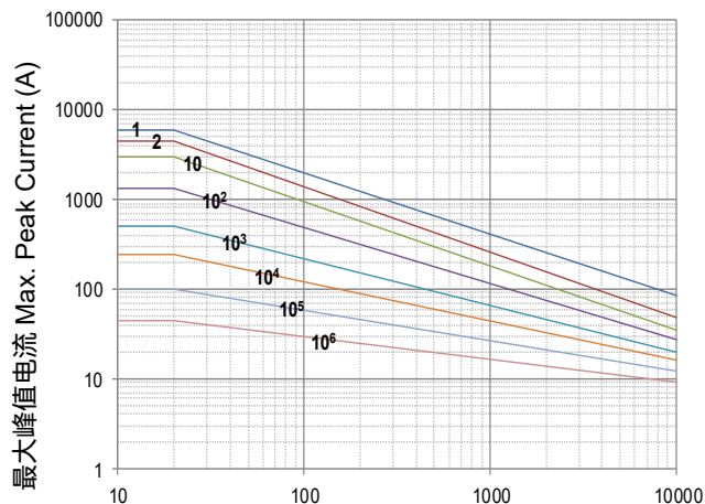
脉冲持续时间 Impulse Duration ( \mu s) SFV25D220KM to SFV25D680KM
