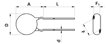
内弯型引线 Inward Crimp
