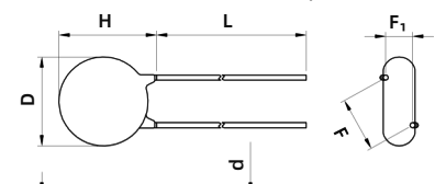
Y型引线 Inline Crimp
