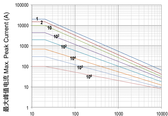
脉冲持续时间 Impulse Duration ( \mu s) SFV25D820K to SFV25D122K
