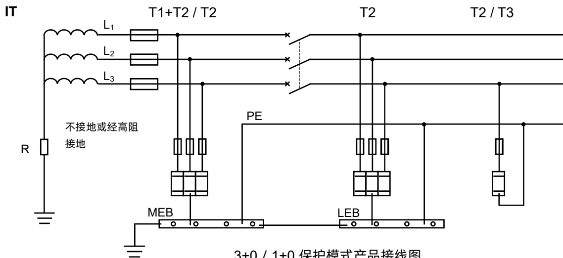
3+0 / 1+0 保护模式产品接线图
