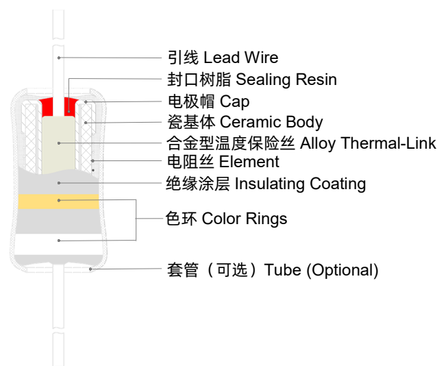
轴向型 Axial Type
